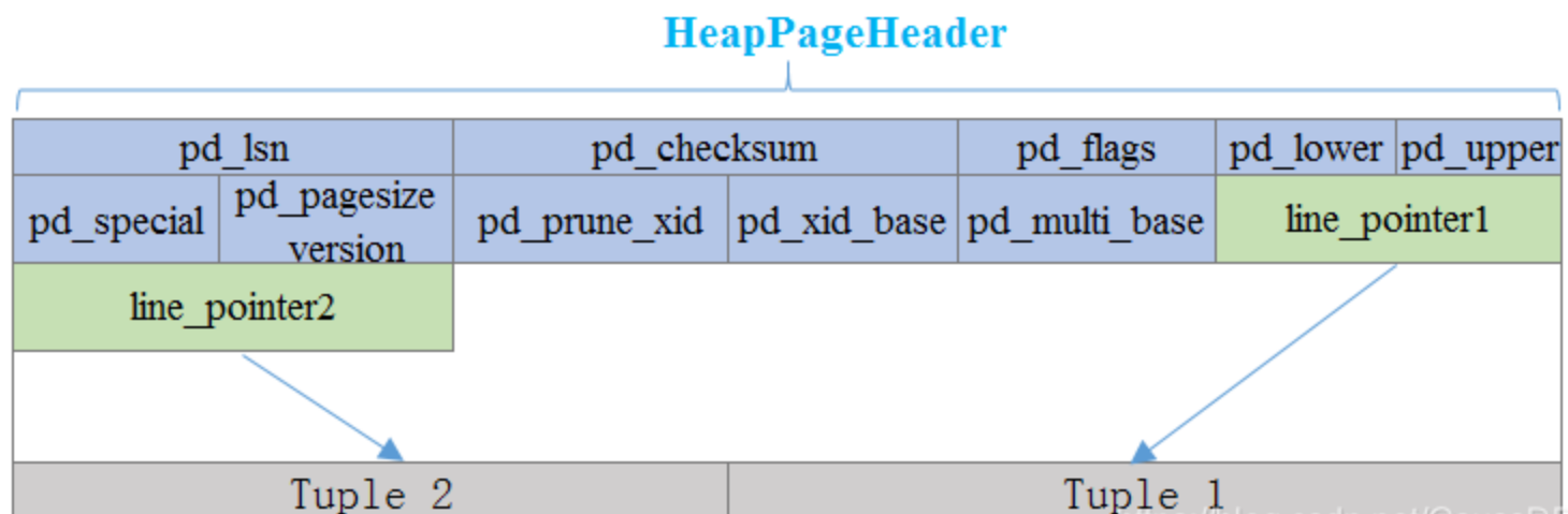
openGauss中采用的astore堆表页面结构示意图
